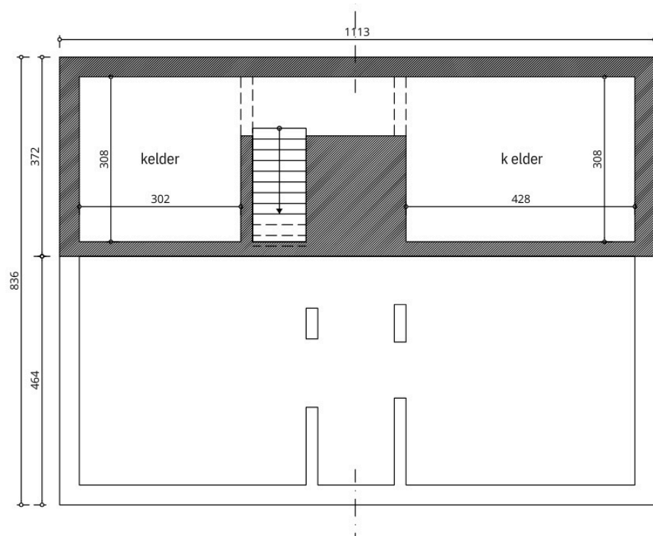
KELDER
