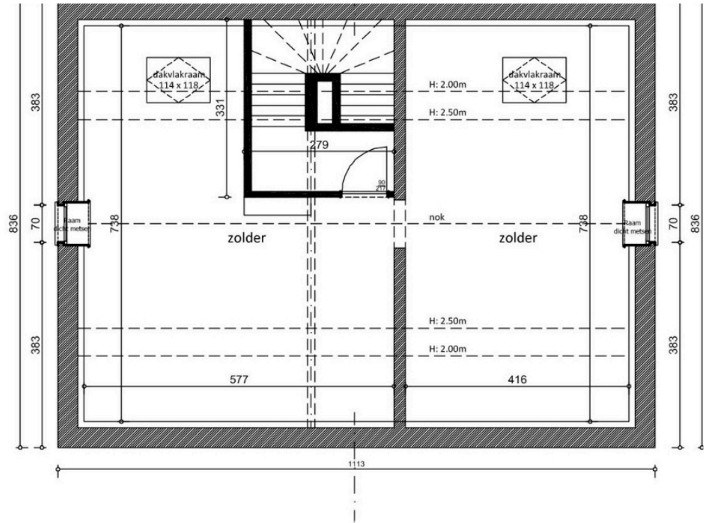
VERDIEPING +2
