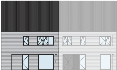
VOORGEVEL
